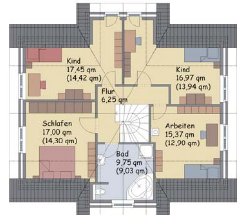
Variante 1 Dachgeschoss
